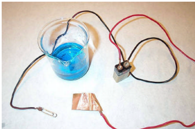
Figura 2. Dispositivo experimental.
