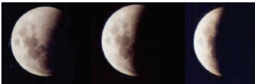
La sombra de la Tierra sobre la Luna durante un eclipse es consecuencia de su forma.
